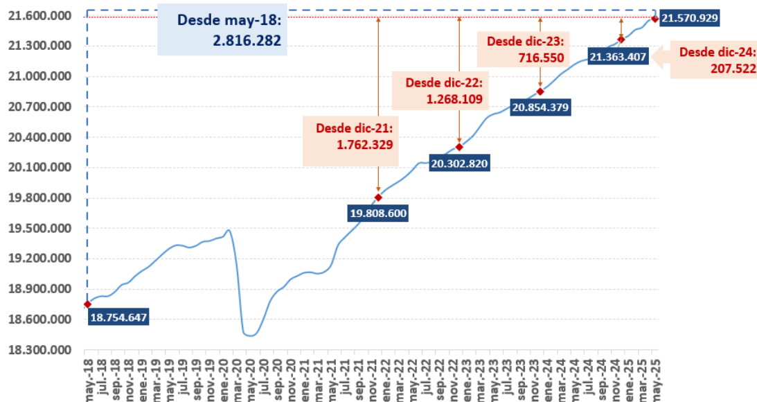
Serie desestacionalizada
